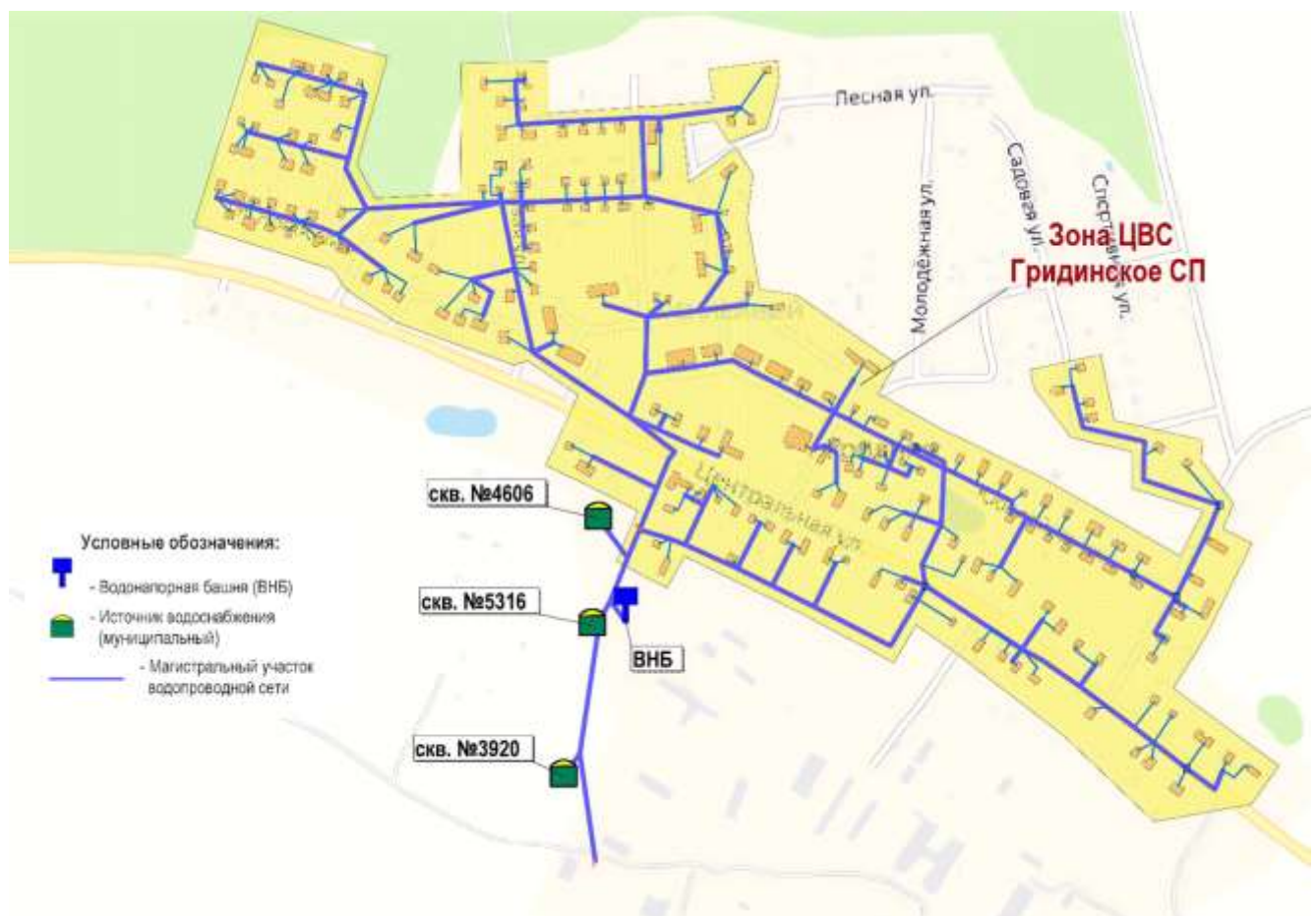
Рис. 1.6. Зона централизованного водоснабжения д.Гридино Гридинского сельского поселения
