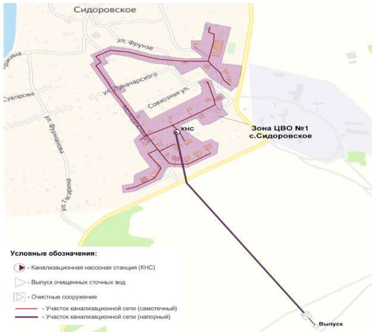
Рис. 1.33. Зона централизованного водоотведения №1 с.Сидоровское Сидоровского сельского поселения
