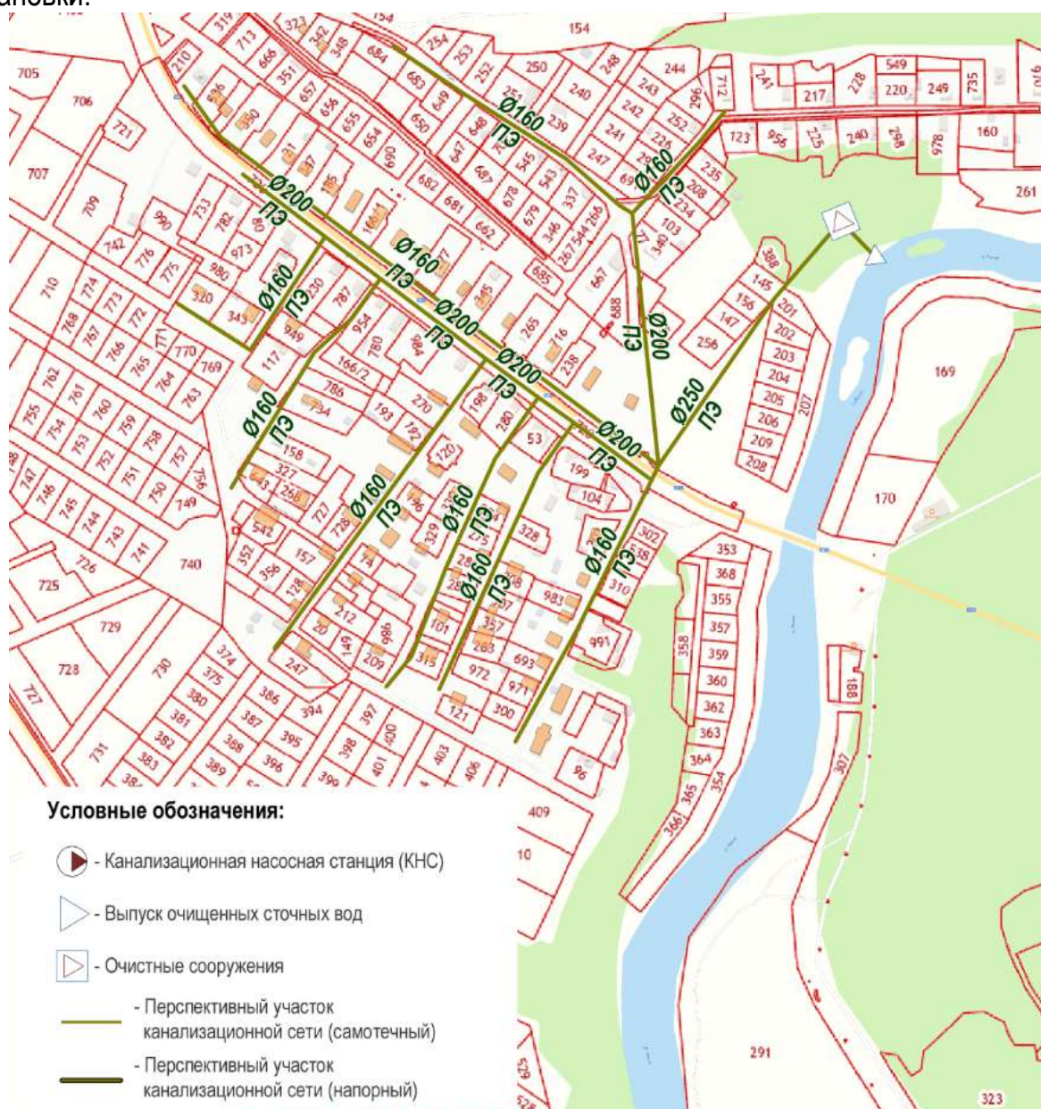
Рис. 4.1. Перспективное водоотведение д.Большое Андрейково
