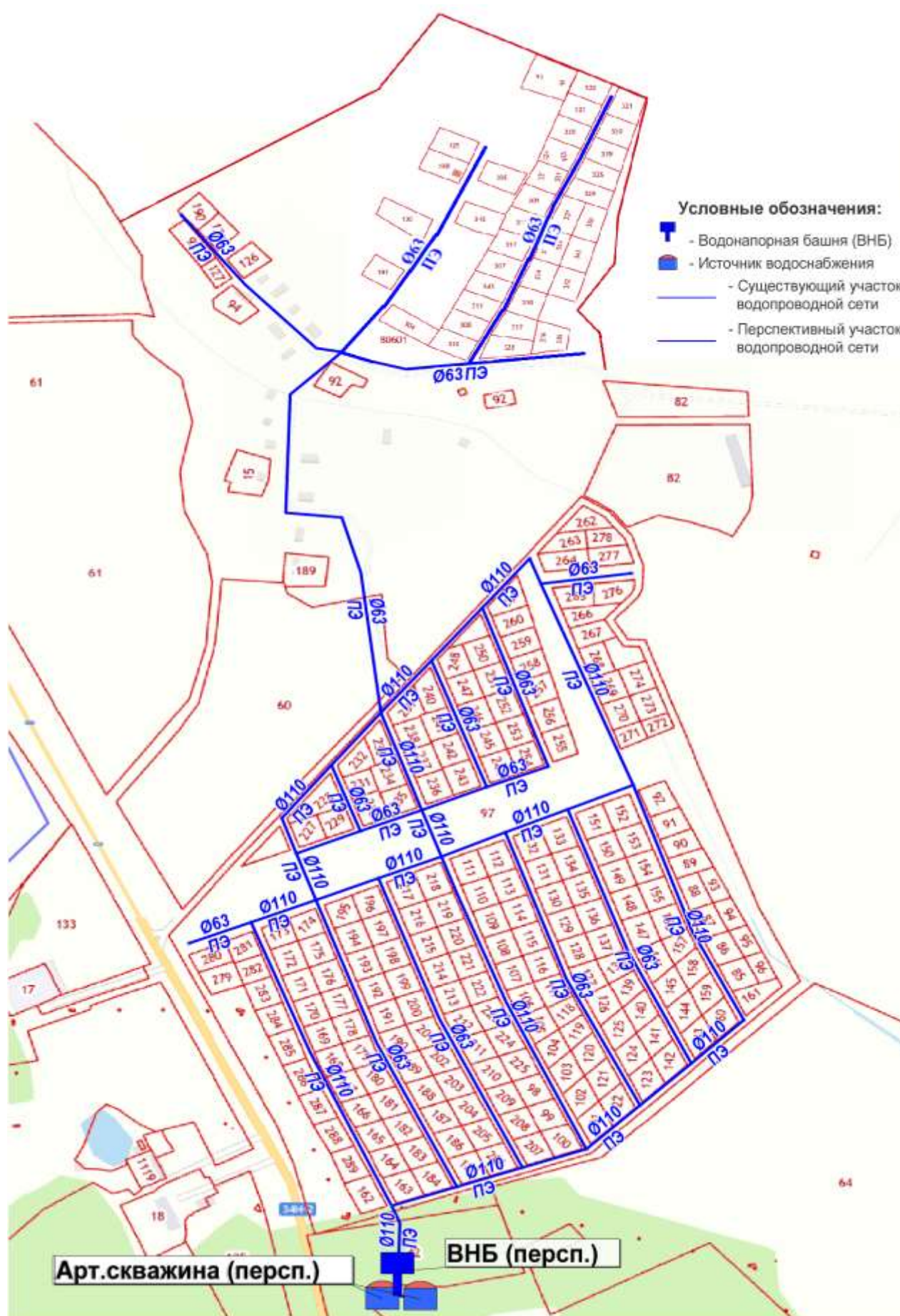
Рис. 4.2. Перспективное водоснабжение в д.Зайцево
