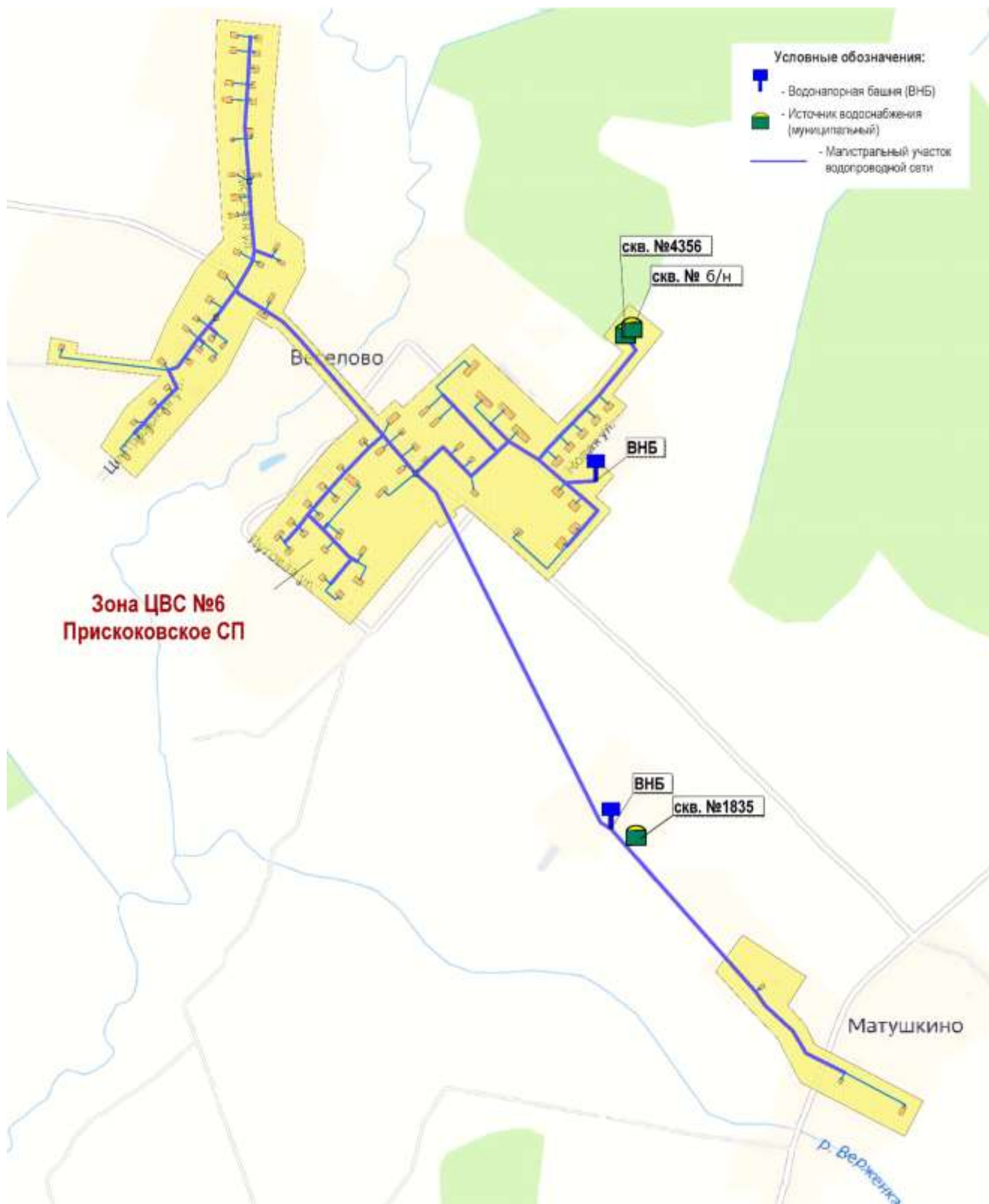
Рис. 1.12. Зона централизованного водоснабжения №6 д.Веселово и д.Матушкино Прискоковского сельского поселения
