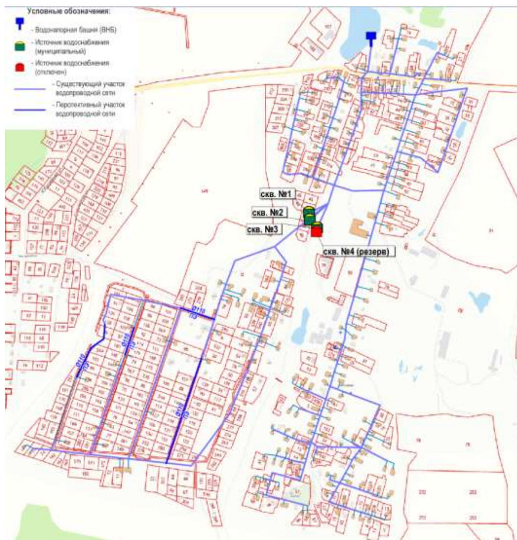
Рис. 4.11. Перспективное водоснабжение в с.Здемирово
