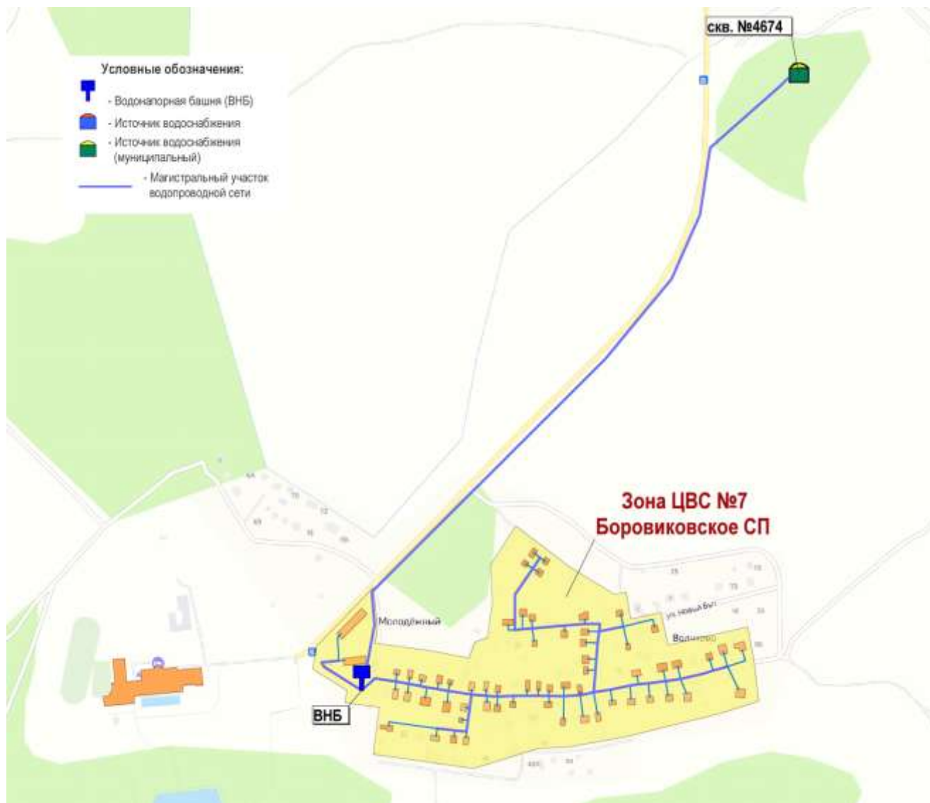
Рис. 1.20. Зона централизованного водоснабжения №7 п.Молодежный и д.Волчково Боровиковского сельского поселения
