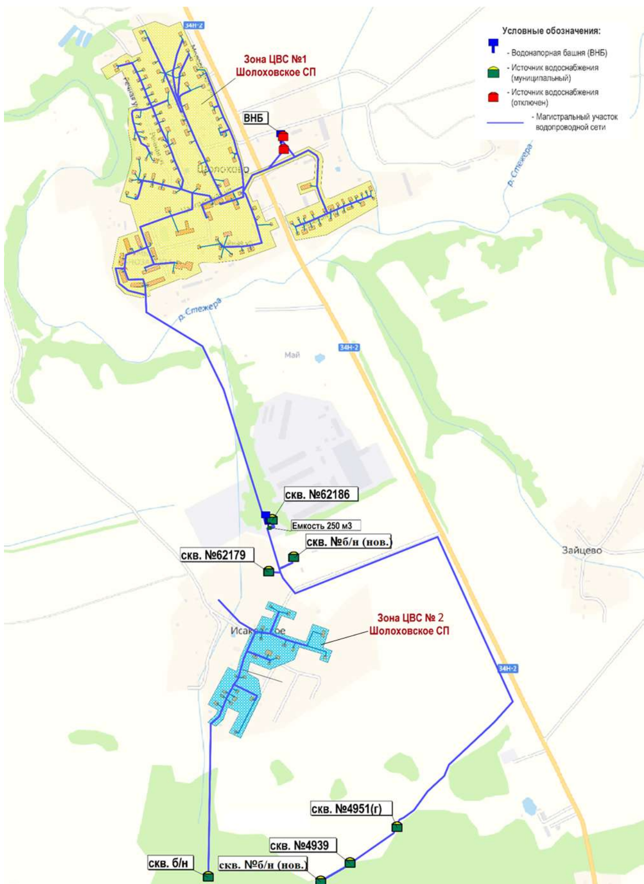
Рис. 1.1. Зоны централизованного водоснабжения №1, №2 д.Шолохово Шолоховского сельского поселения
