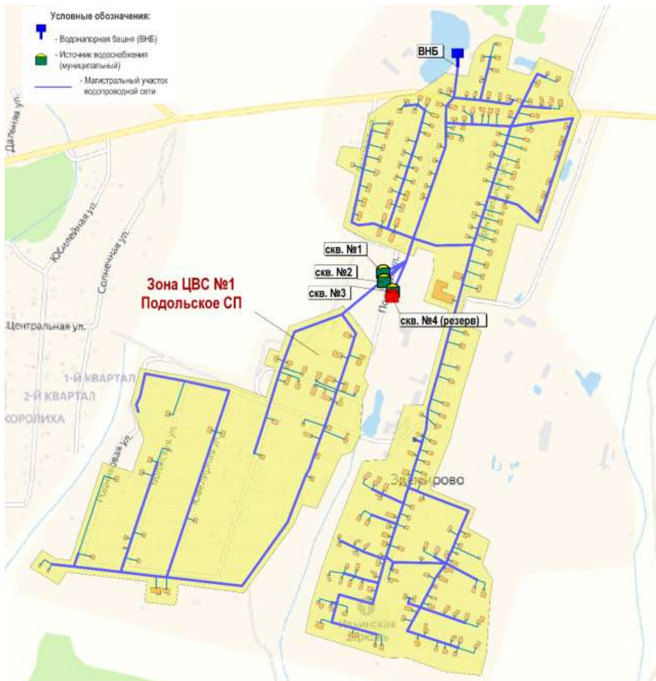
Рис. 1.36. Зона централизованного водоснабжения №1 с.Здемирово Подольского сельского поселения
