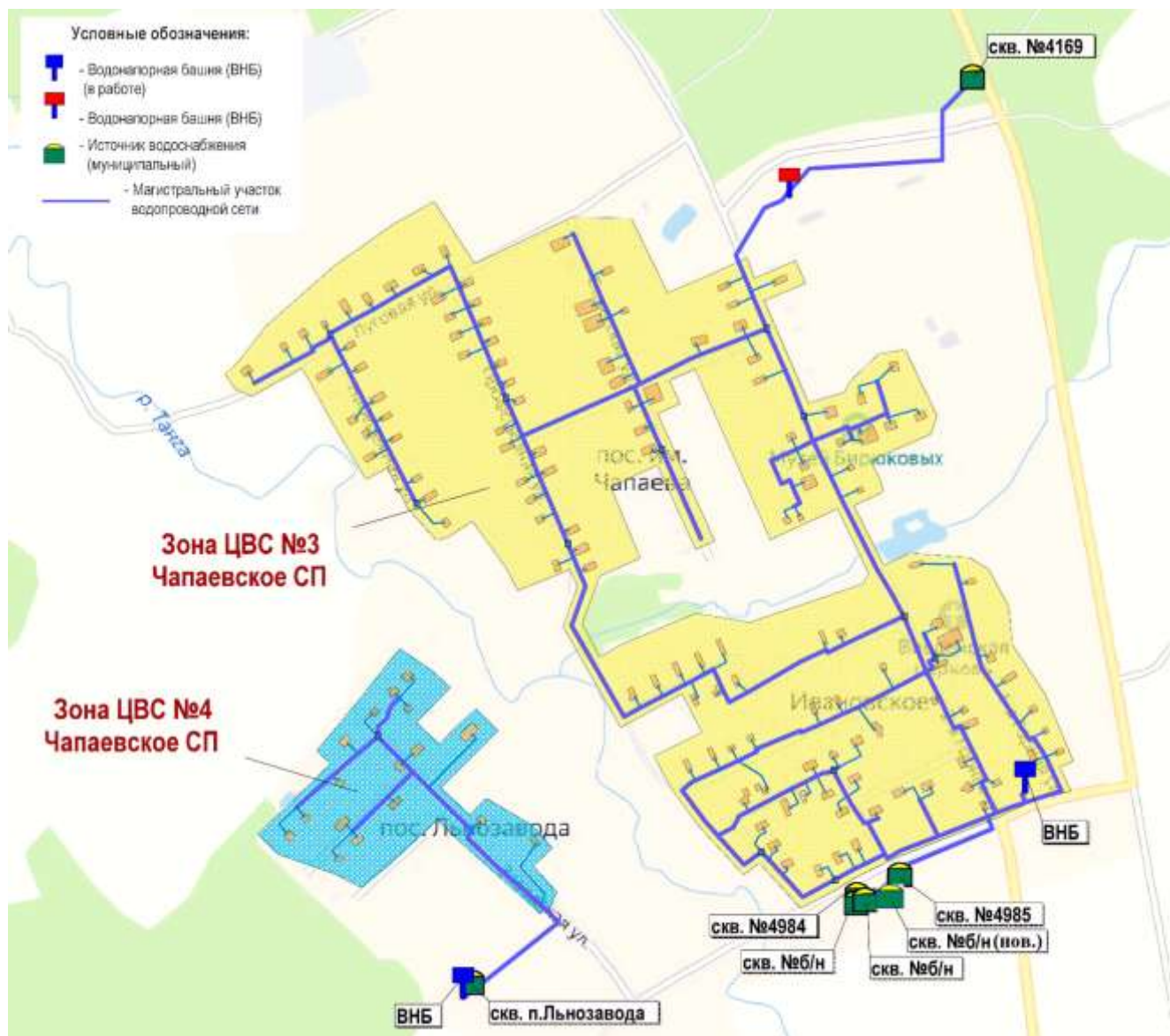
Рис. 1.25. Зоны централизованного водоснабжения №3 п.им. Чапаева и д.Ивановское и №4 п.Лынозавода Чапаевского сельского поселения
