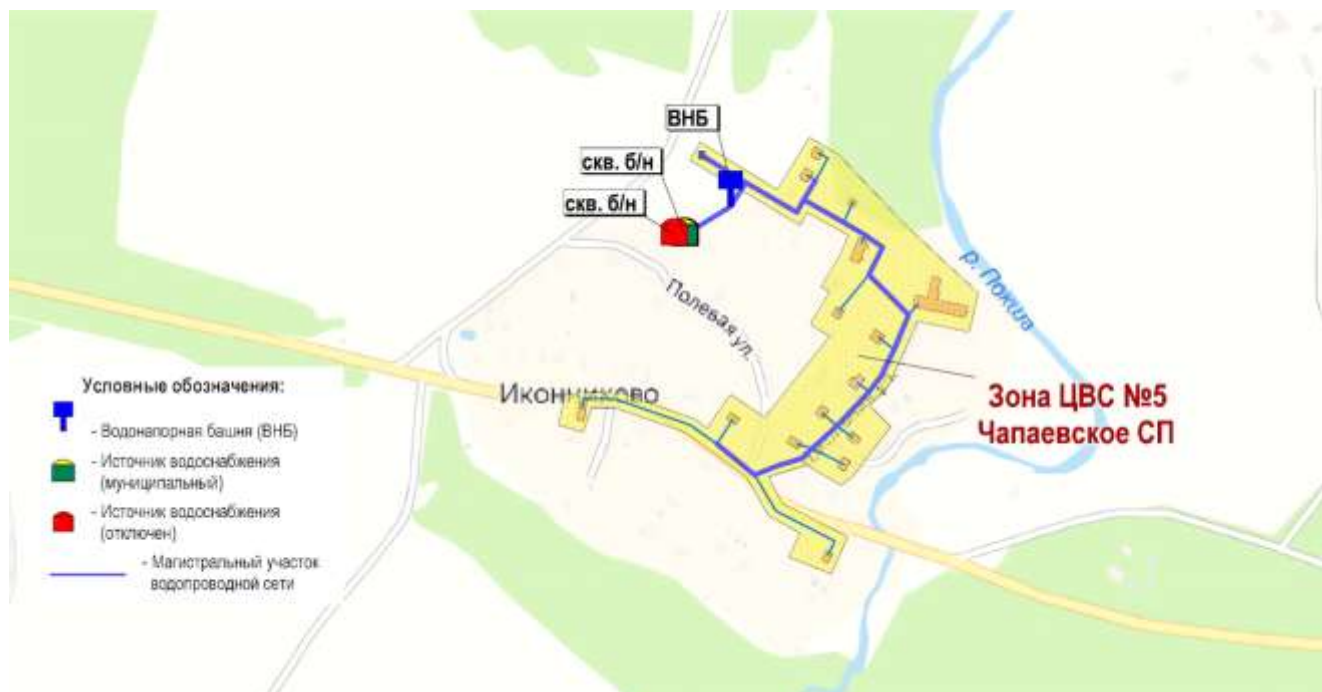
Рис. 1.26. Зона централизованного водоснабжения №5 д.Иконниково Чапаевского сельского поселения
