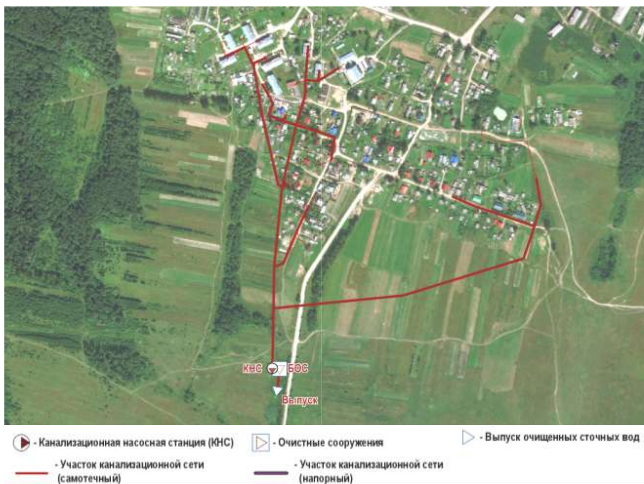
Рис. 1.13. Расположение очистных сооружений д.Ченцы
