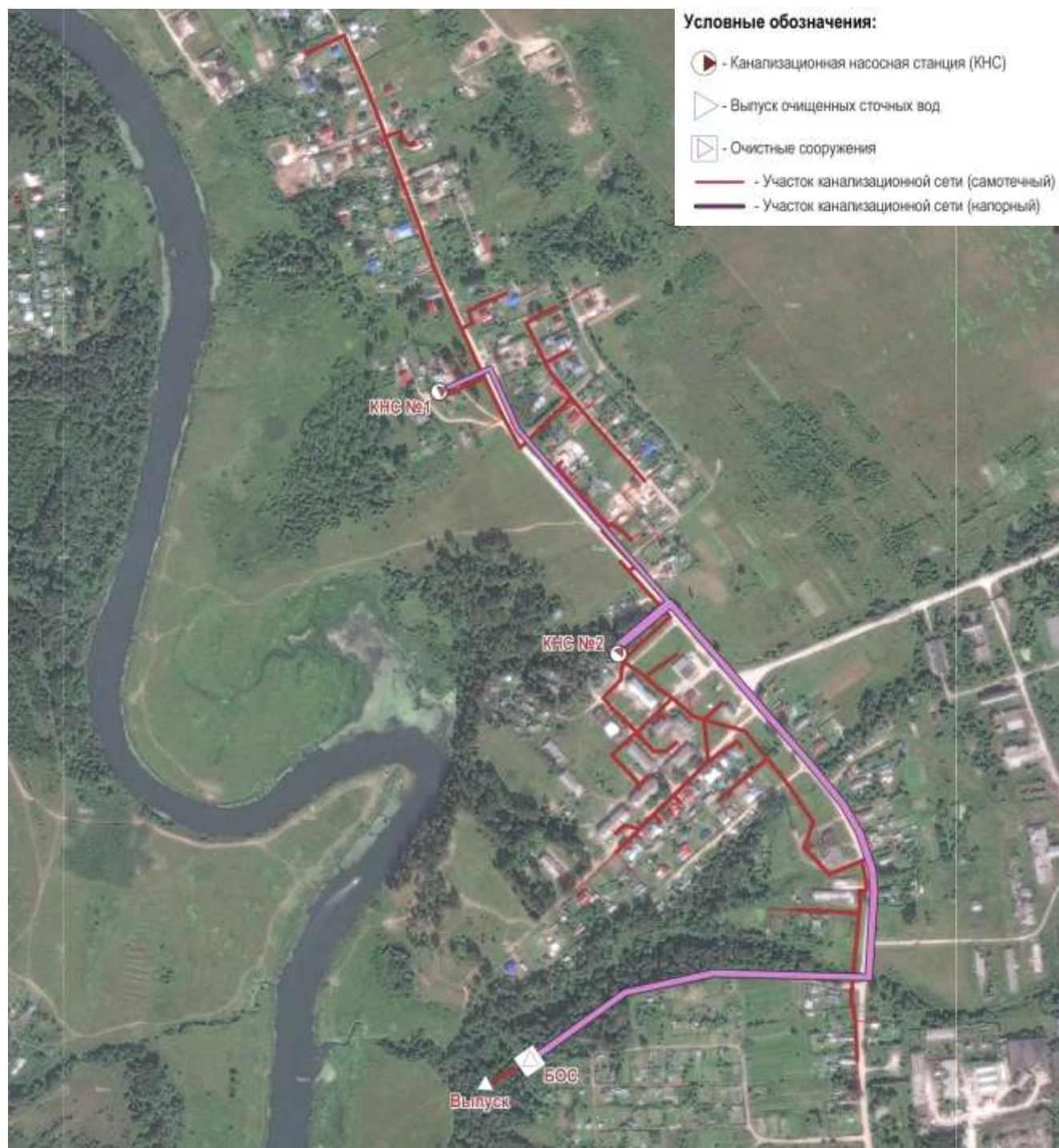
Рис. 1.8. Расположение очистных сооружений д.Боровиково
